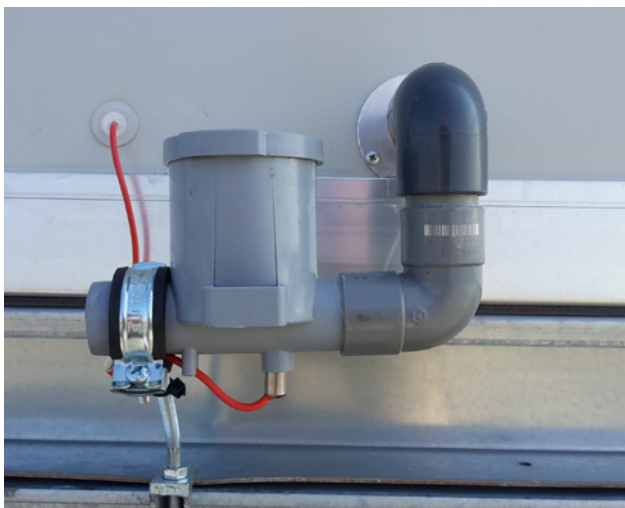
Sifon op de unit.
