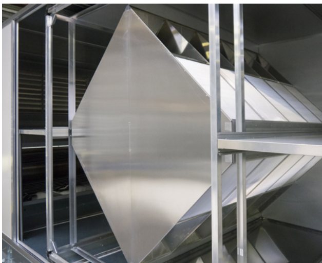
Tegenstroomplatenwisselaar in de unit (tijdens opbouw).
